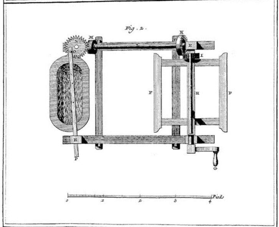
Soierie, Tirage de la Soie et Plan du Tour de Piémont.
