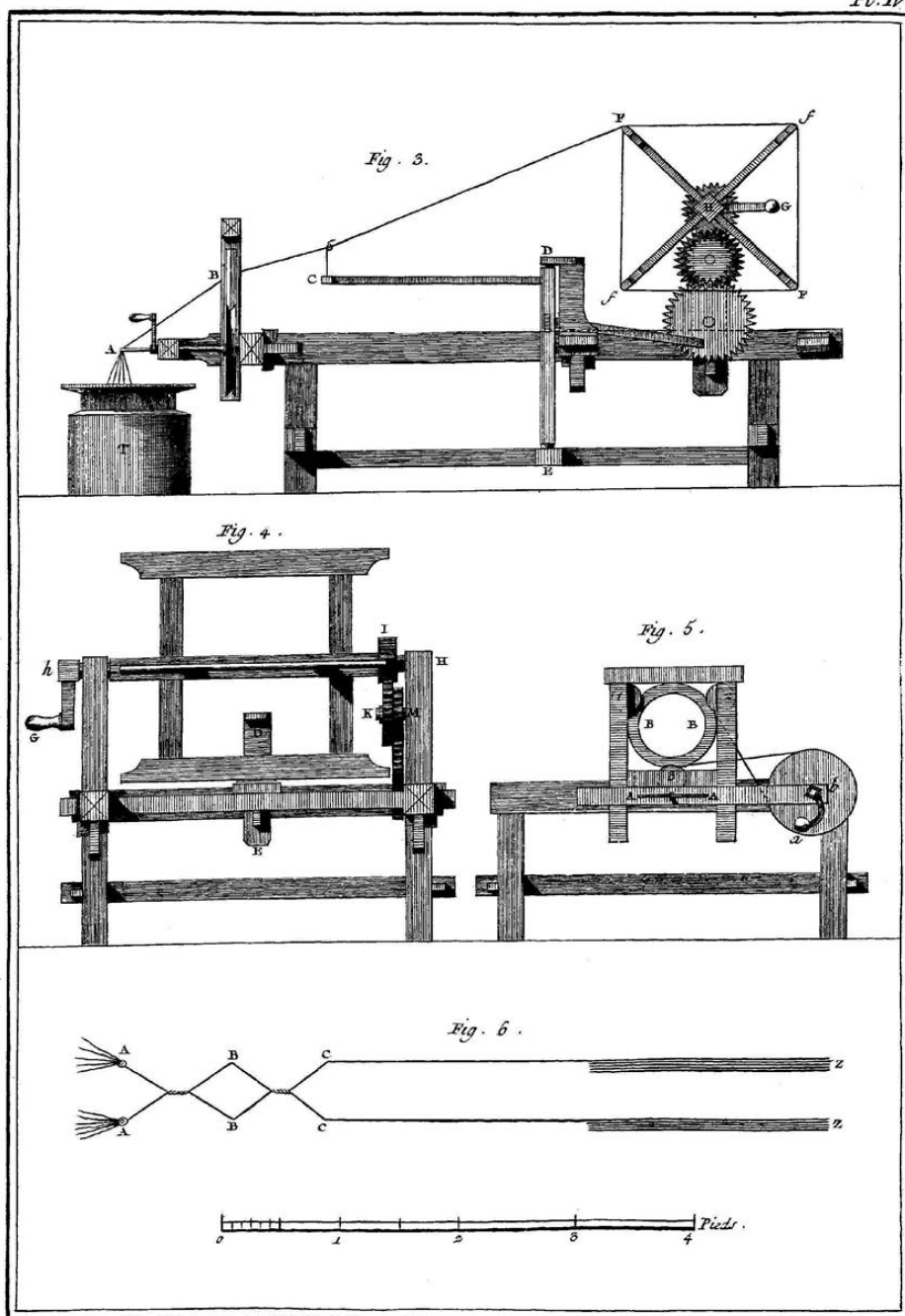
Soierie, Développement du Tour de M r de Vaucanson.
