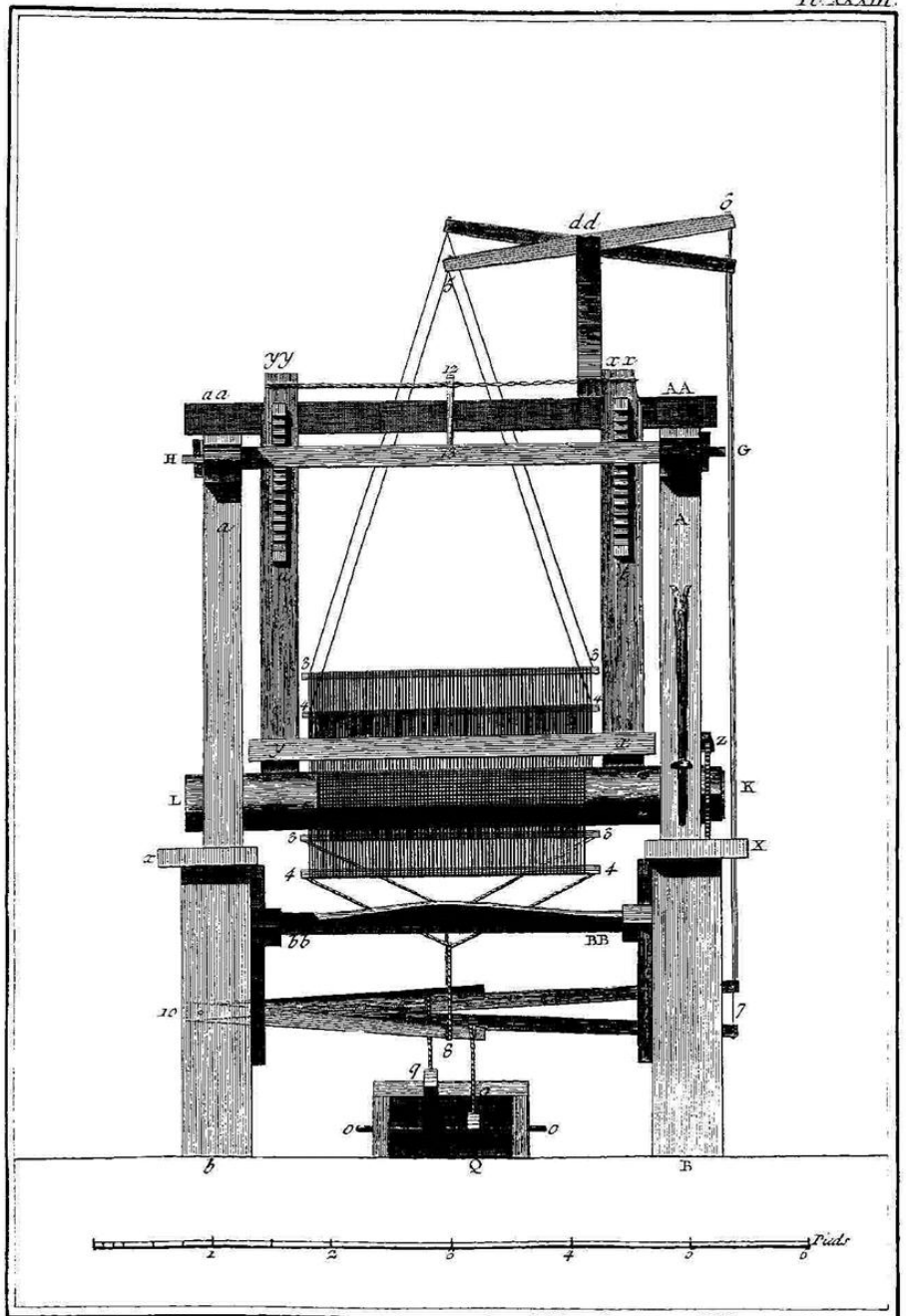
Soierie, Élévation Géométrale de la partie antérieure du métier pour fabriquer les étoffes unies, comme Taffetas, satin, et serge
